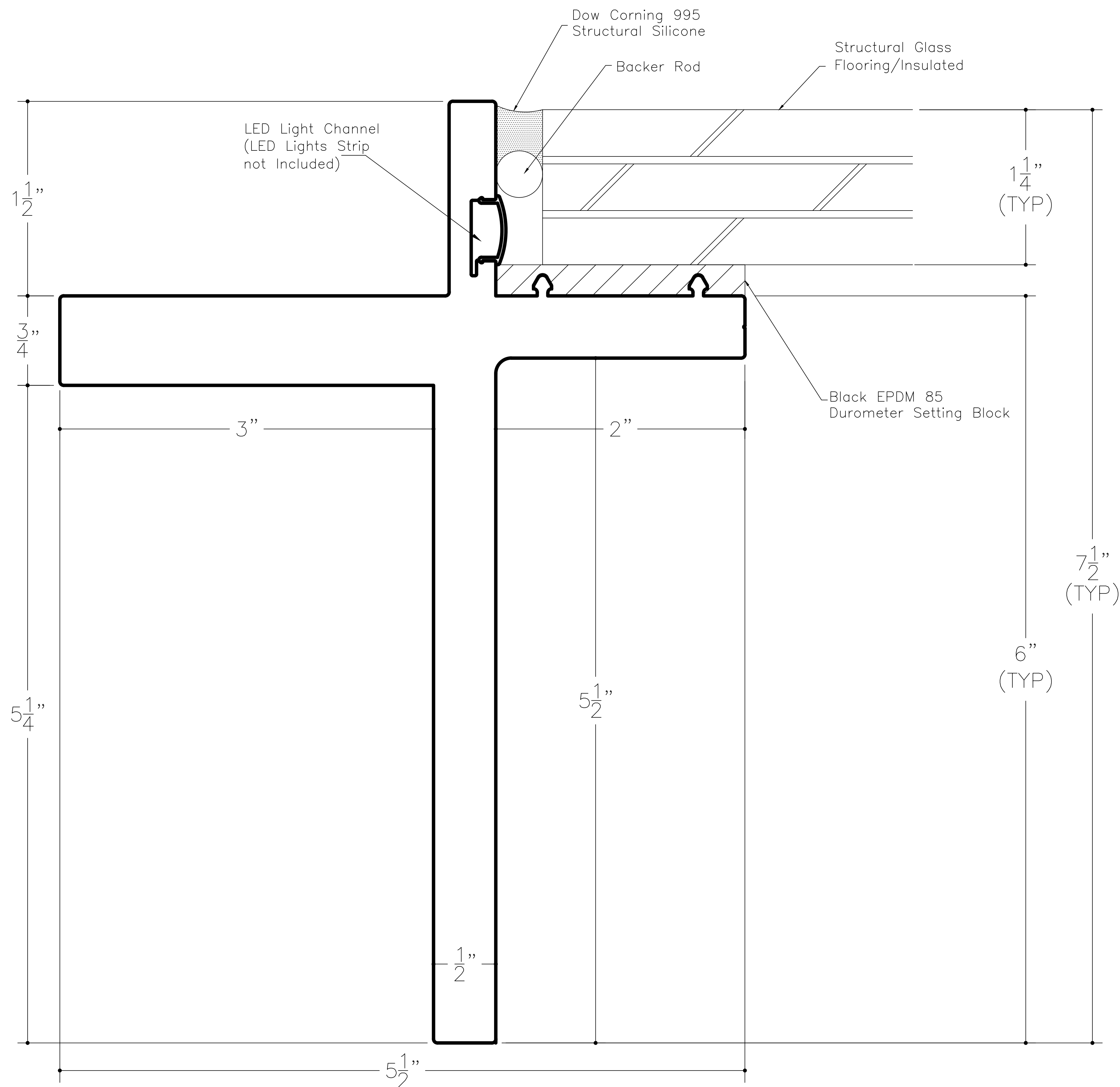
SkyFloor® Non Thermal Perimeter
